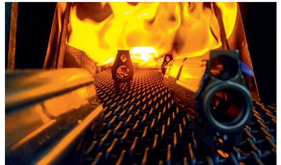
Le boîtier culasse lors de la fabrication dans le four.
